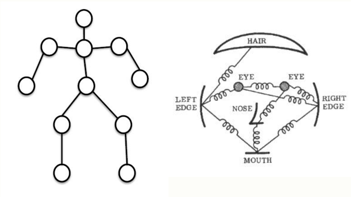
图结构模型
