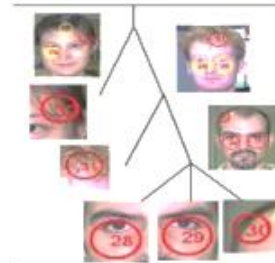
与或图模型
