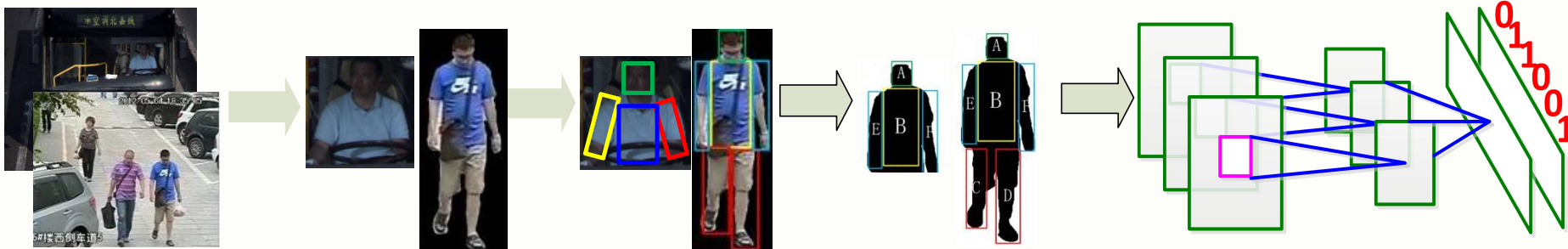
多部件特征
