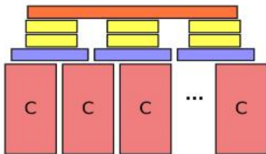
4) Local Pooling
