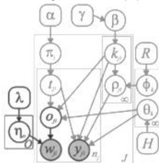
非参贝叶斯
