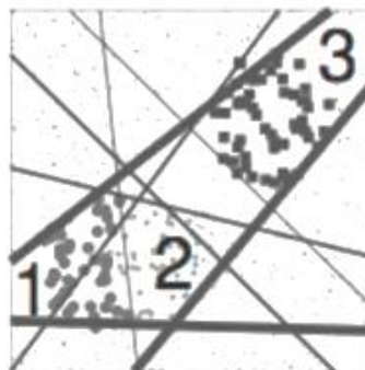
提升(Boosting)
