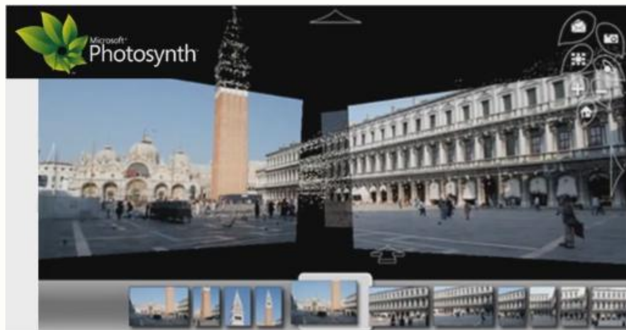
图像拼接
